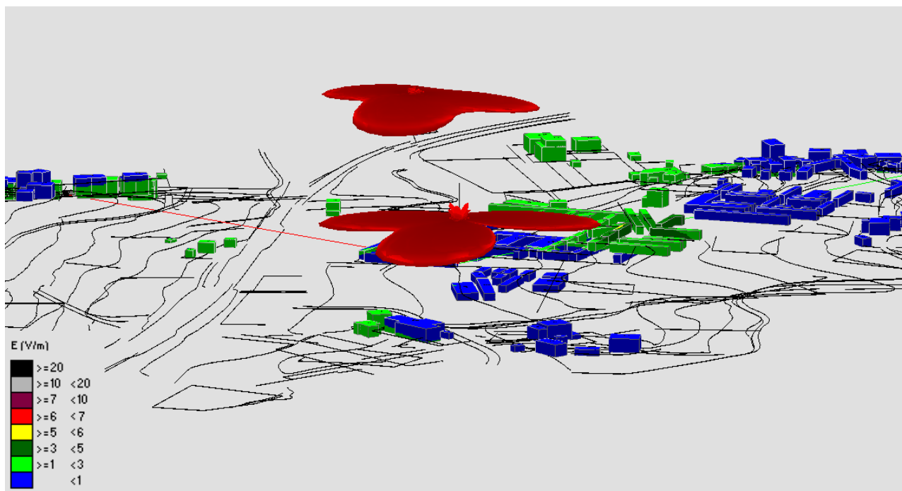
Fig. 284 Impatto elettromagnetico – Zona Area Cimitero Strada Vallelunga – Vista Laterale 1
