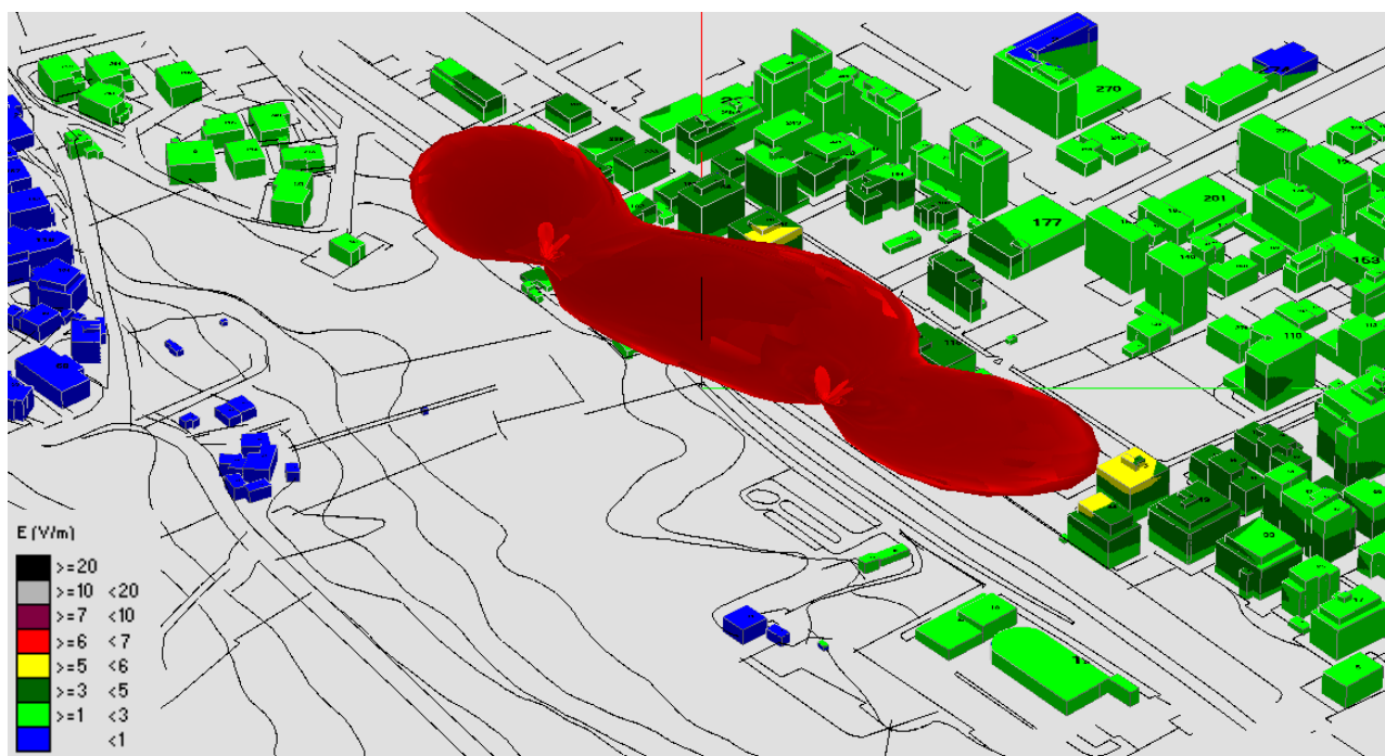
Fig. 37 Impatto elettromagnetico – Zona Via Caravaggio – 0°/Nord
