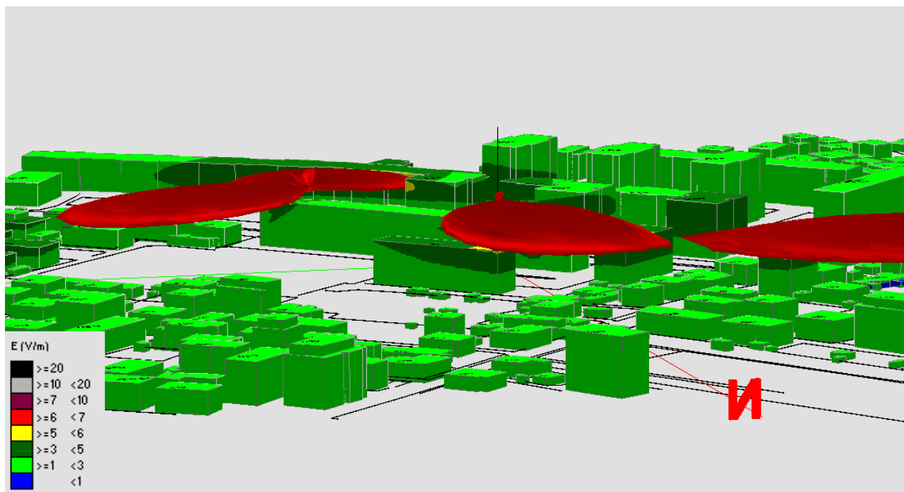
Fig. 164 Impatto elettromagnetico – Zona Area case Popolari Via Lago di Capetrano – Vista Laterale 1
