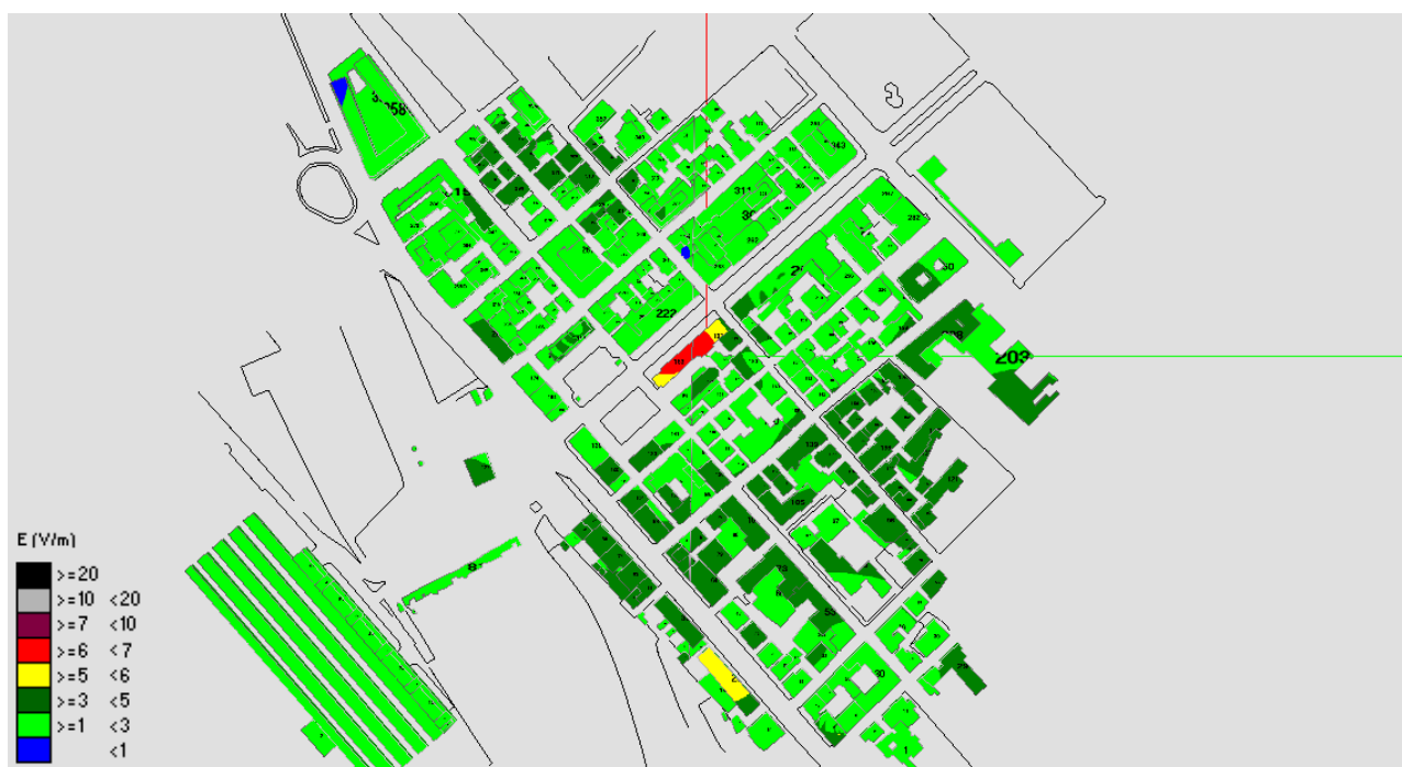
Fig. 103 Impatto elettromagnetico – Zona Piazza Sacro Cuore – Vista dall'alto
