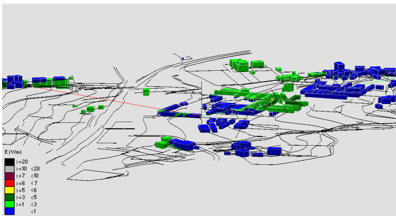
Fig. 285 Impatto elettromagnetico – Zona Area Cimitero Strada Vallelunga – Vista Laterale 2
