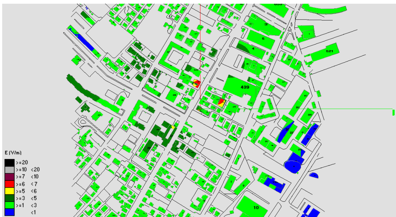
Fig. 213 Impatto elettromagnetico – Zona Via Fortore – Vista dall'alto
