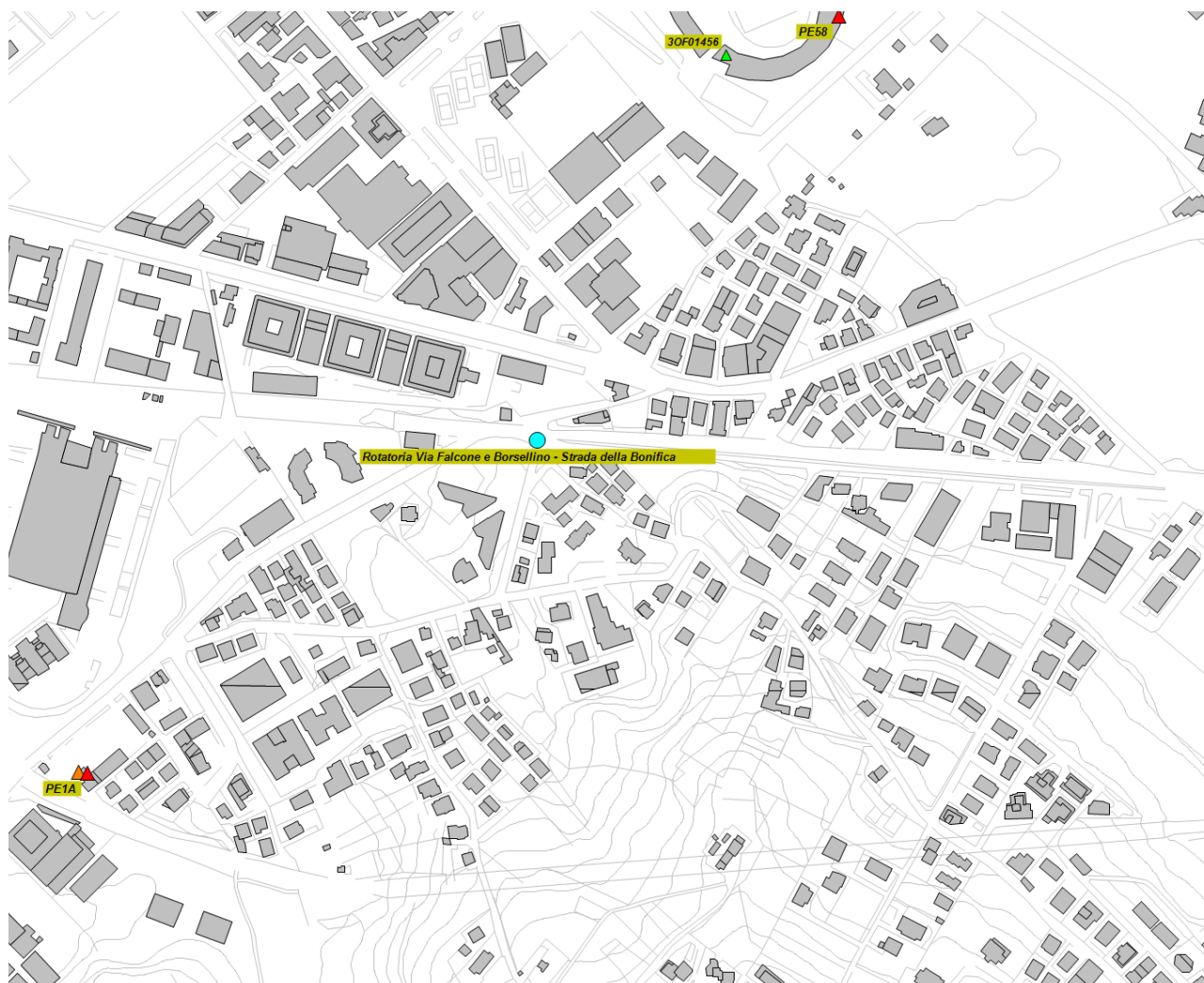
Fig. 286 Impianti considerati nella Zona Rotat. V Falcone e Borsellino-Stda della Bonifica
