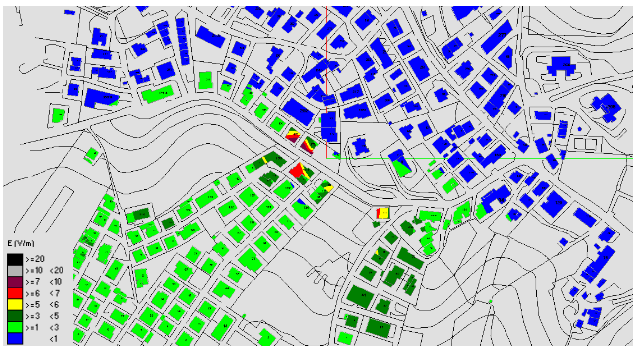
Fig. 23 Impatto elettromagnetico – Zona Via di Colle Scorriano – Vista dall'alto
