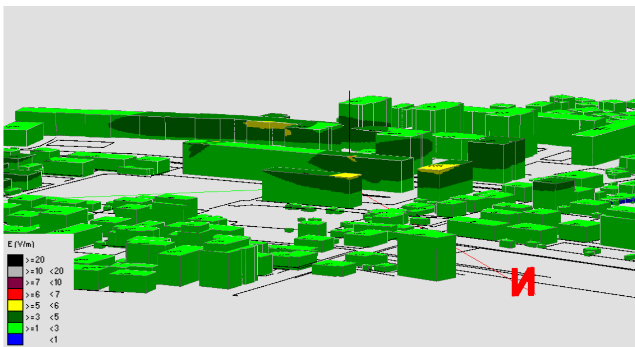
Fig. 165 Impatto elettromagnetico – Zona Area case Popolari Via Lago di Capetrano – Vista Laterale 2
