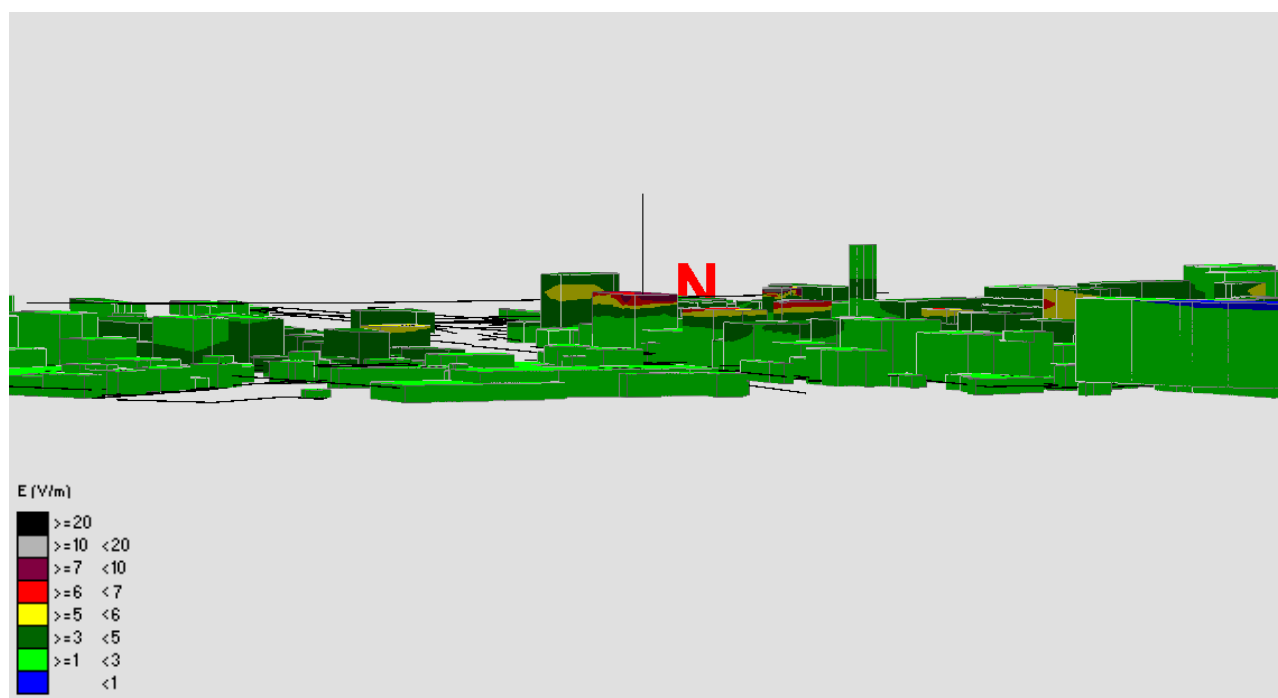
Fig. 135 Impatto elettromagnetico – Zona Via dei Bastioni - Via Saline – Vista Laterale 2
