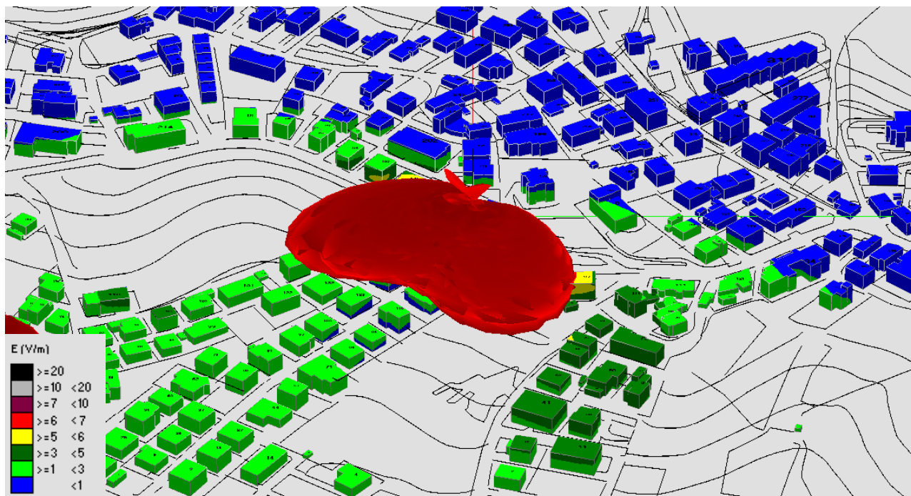
Fig. 22 Impatto elettromagnetico – Zona Via di Colle Scorriano – 0°/Nord
